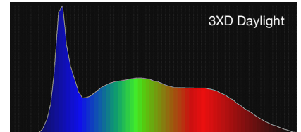
EBU : TLCI-2012
